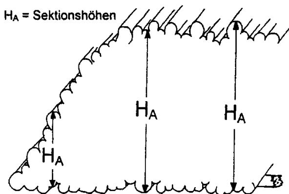
Abbildung 10: Methodik der Sektionshöhenmessung
