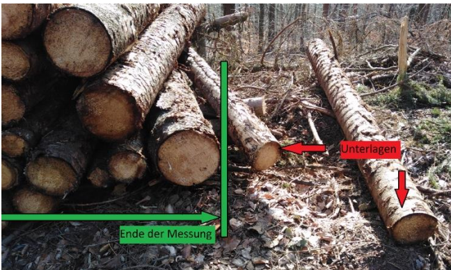
Abbildung 9: Poltergesamtlänge Sektionsraummaß - Beginn/Ende der Messung
